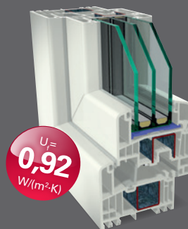
Úzký rám s křídlem, vhodný pro pasivní domy, v souladu se směrnici iřt
